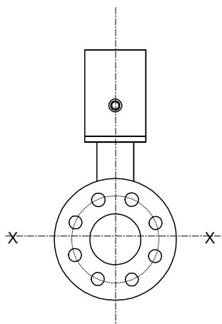
Рисунок 3 Варианты установки ППР (расходомера)
